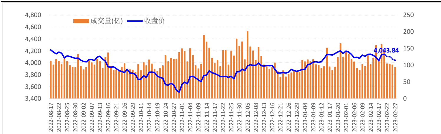
图4: 沪深300走势图
