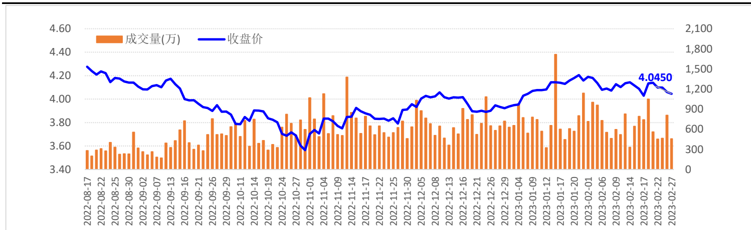
图3: SZ300ETF走势图
