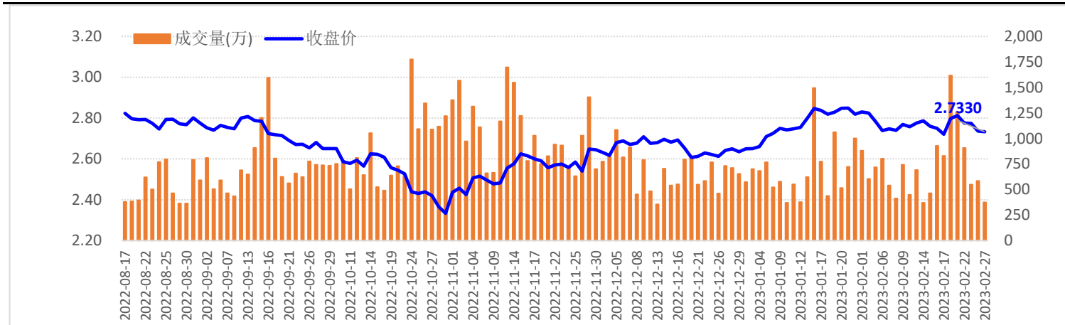
图2 SH300ETF走势图
