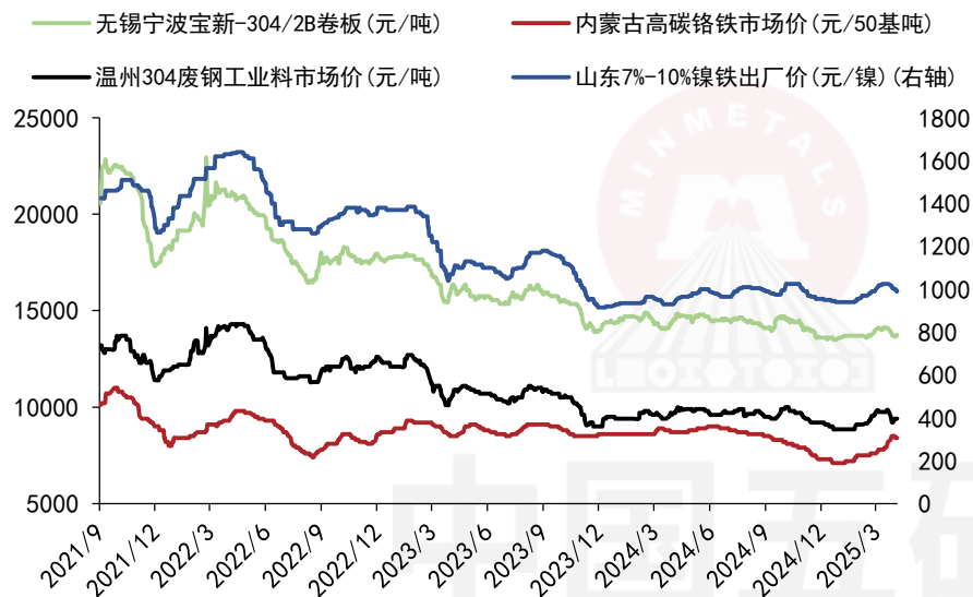
图1：不锈钢链现货价格(元/吨) (元/镍点)
