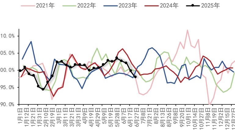
图195：柴油产销率（%）
