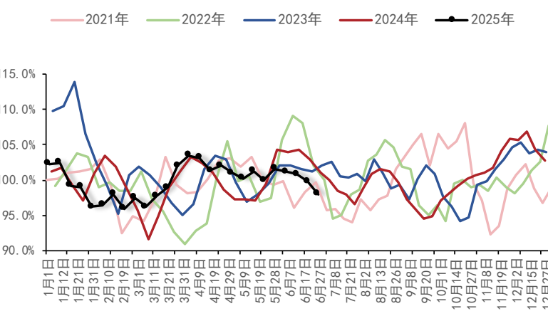
图191：汽油产销率（%）
