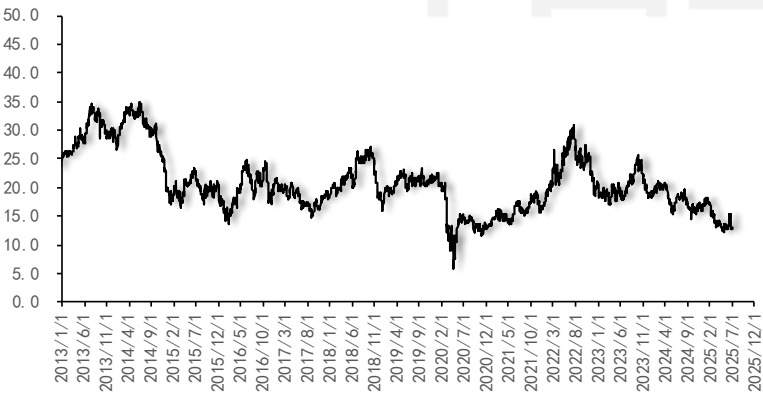
图6：油铜比（%）
