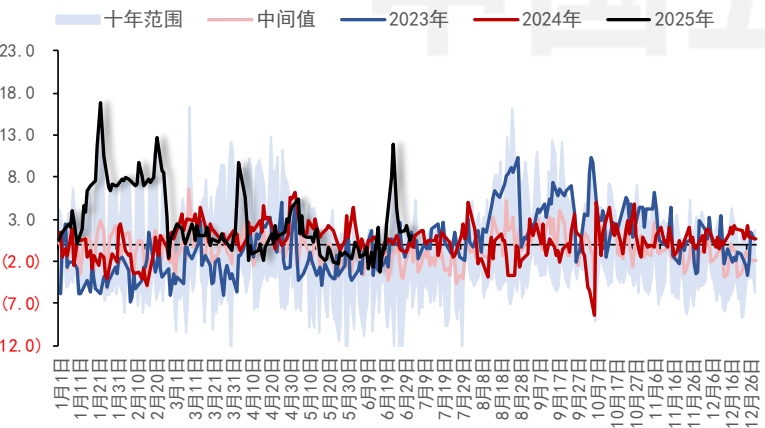
图32: INE/Brent ($/桶)
