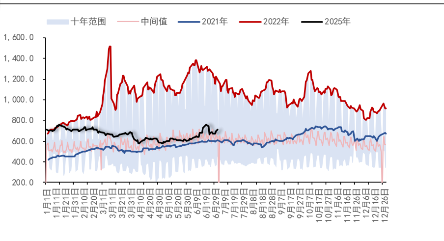
图37：LGO/RB（$/桶）
