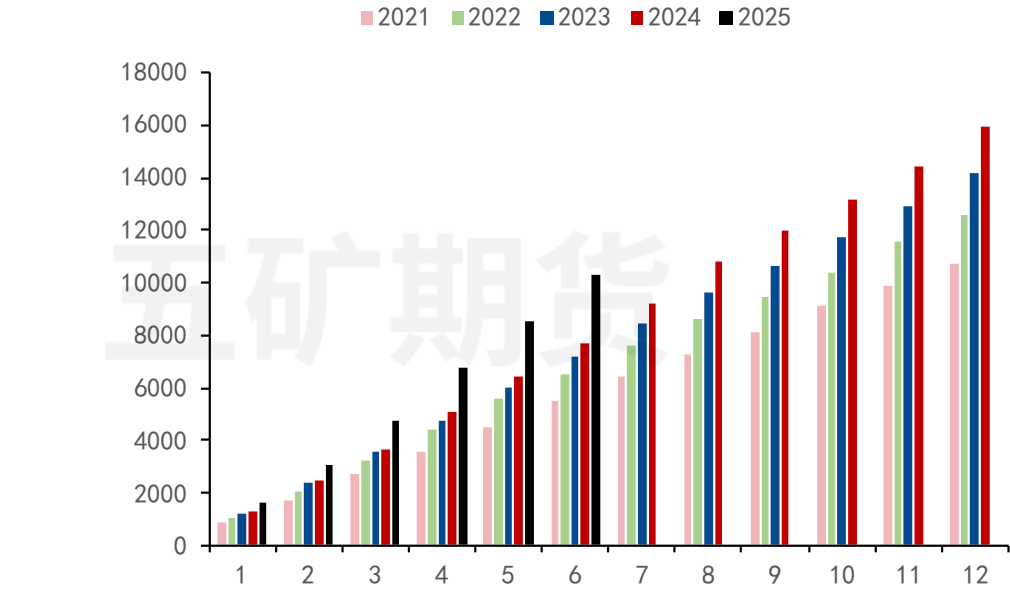
图10：中国铝土矿累计进口（万吨）
