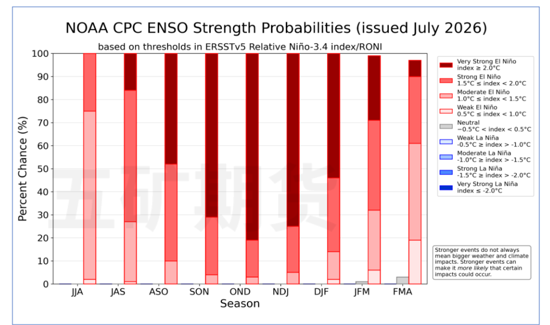
图22：厄尔尼诺强度概率预测（%）
