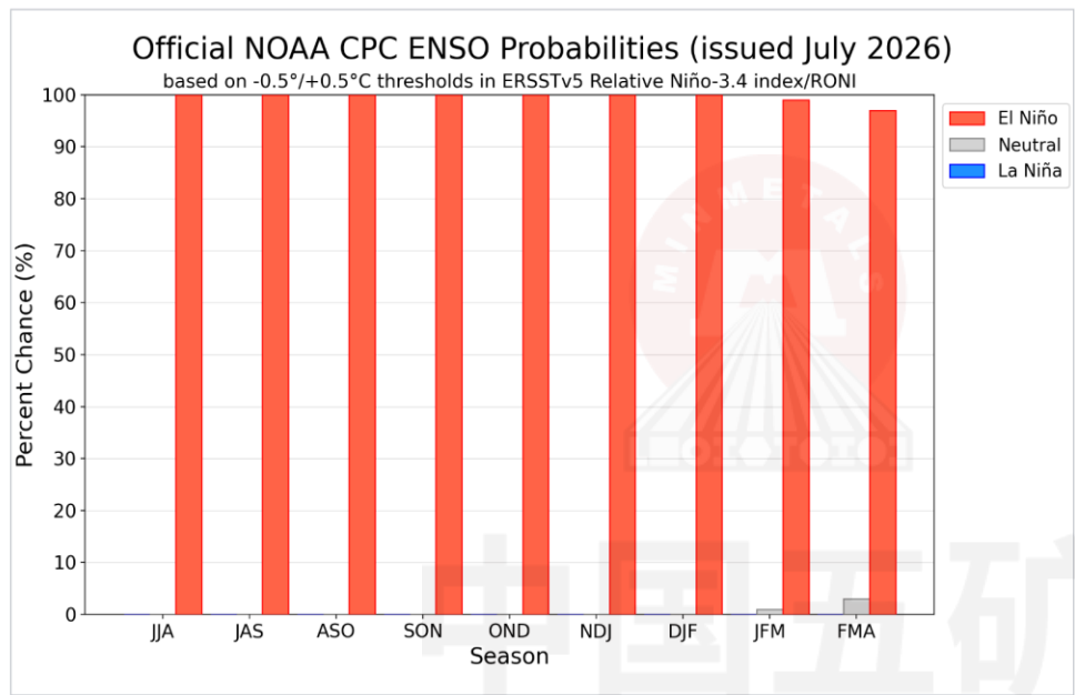
图21：厄尔尼诺发生概率预测（%）
